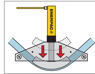
▲ Работа «Одношагового трубогиба».
