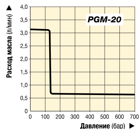
ЗАВИСИМОСТЬ РАСХОДА МАСЛА ОТ ДАВЛЕНИЯ
